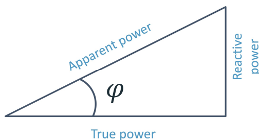
Fig. B.7.1.1 Power triangle
